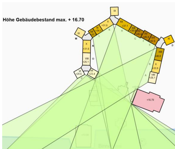
Bestand 5. Geschoss
