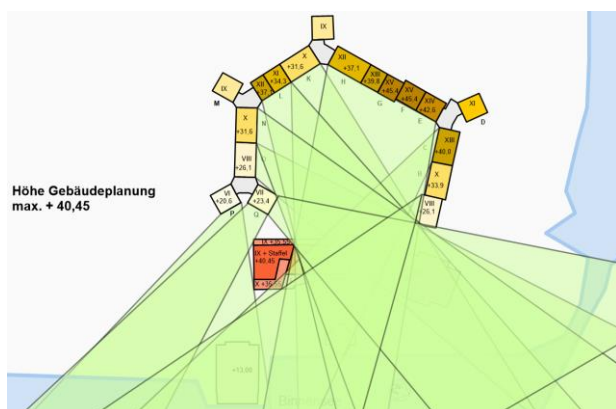
Planung 6. Geschoss
