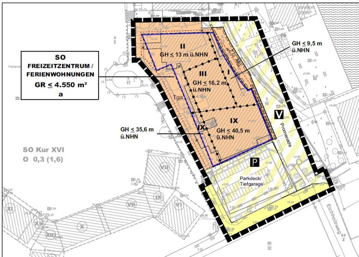
Abbildung 3: B-Plan-Entwurf (Stand 07.08.2019)
