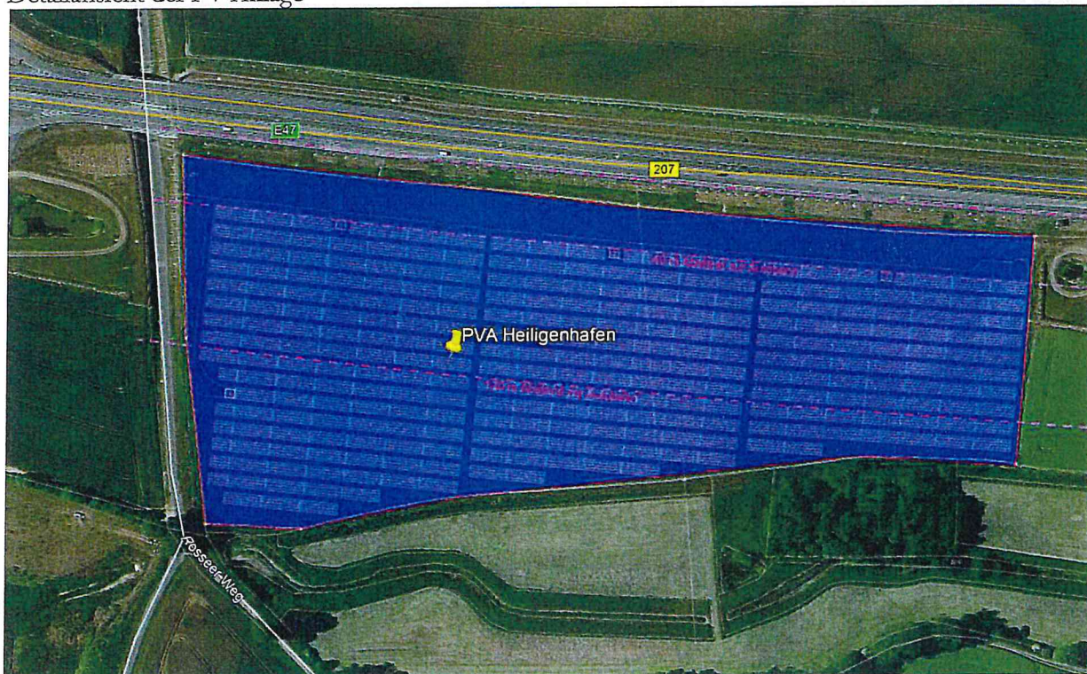
Bild 2.1.3: Detailansicht der PV Anlage (Quelle: Google Earth/SolPEG)
