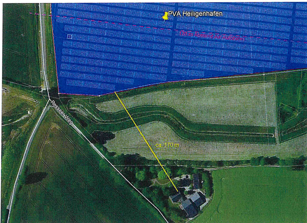
Bild 2.2.1: PV Anlage und Umgebung (Quelle: Google Earth/SolPEG)
