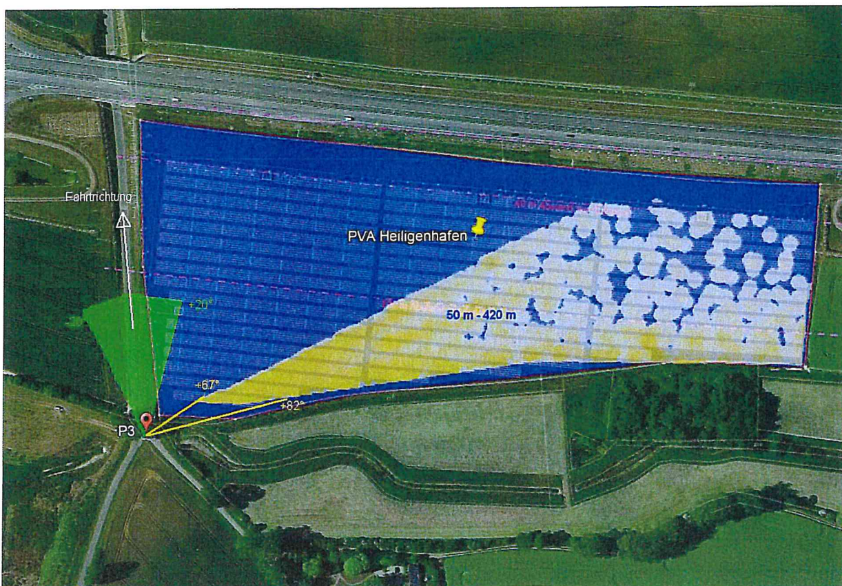
Bild 4.4.2: Simulation am Messpunkte P3 (Quelle: Google Earth/SolPEG)
