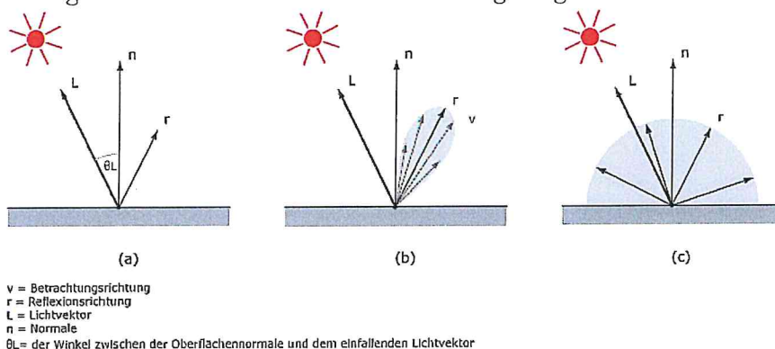
Bild 3.2.4: Diffuse Reflexion von unterschiedlichen Moduloberflächen (© Jürgen Hagler)
