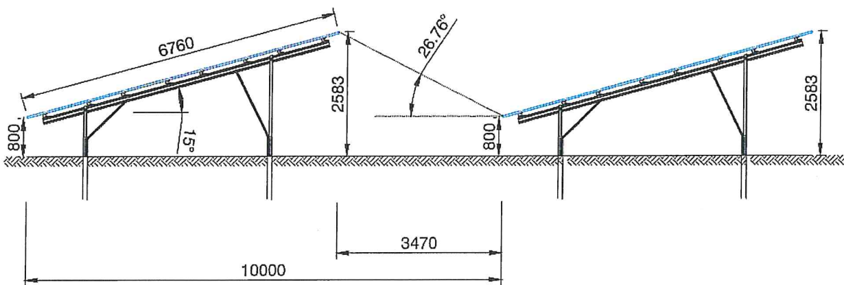
Bild 3.4.1: Skizzen der Modulkonstruktion (Quelle: Auftraggeber)
