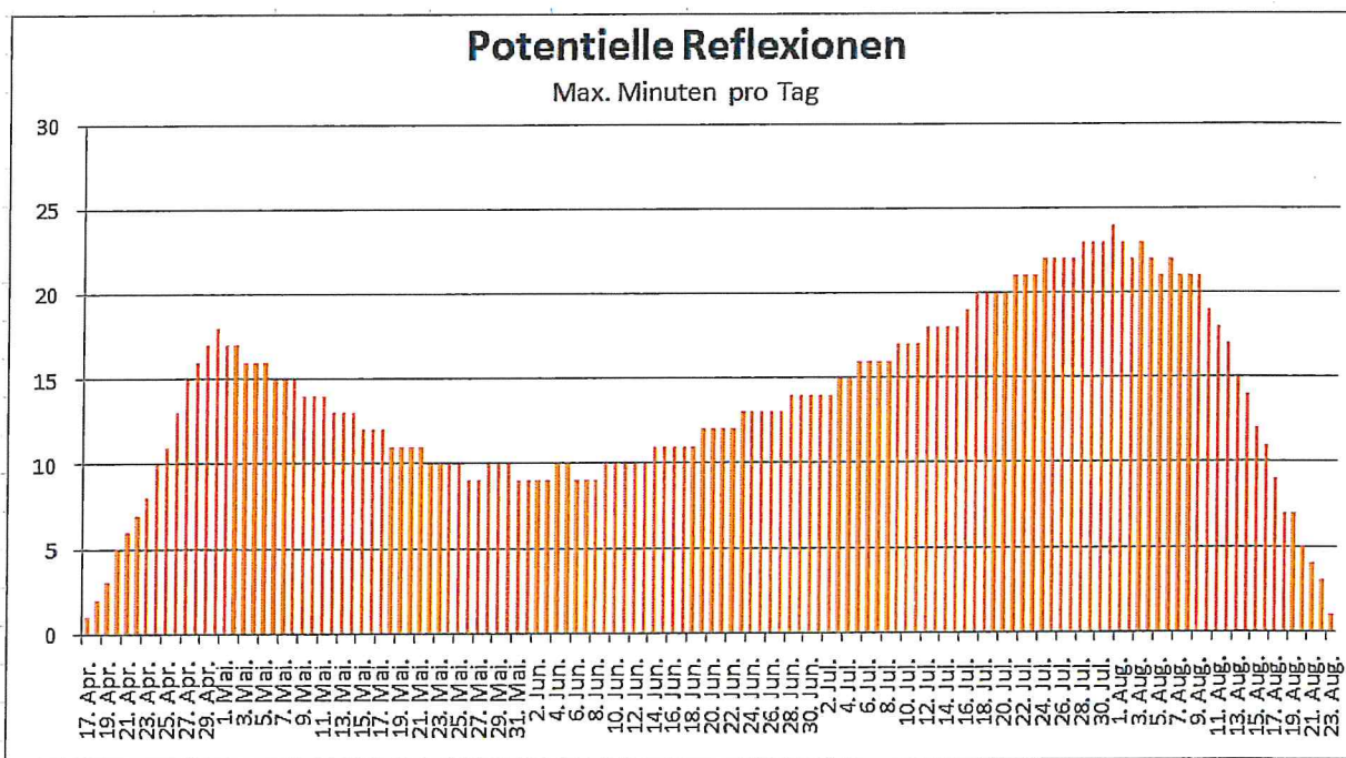
Bild 4.4.1: Reflexionen pro Tag im Jahresverlauf (Quelle: Simulationsergebnisse, aufbereitet)
