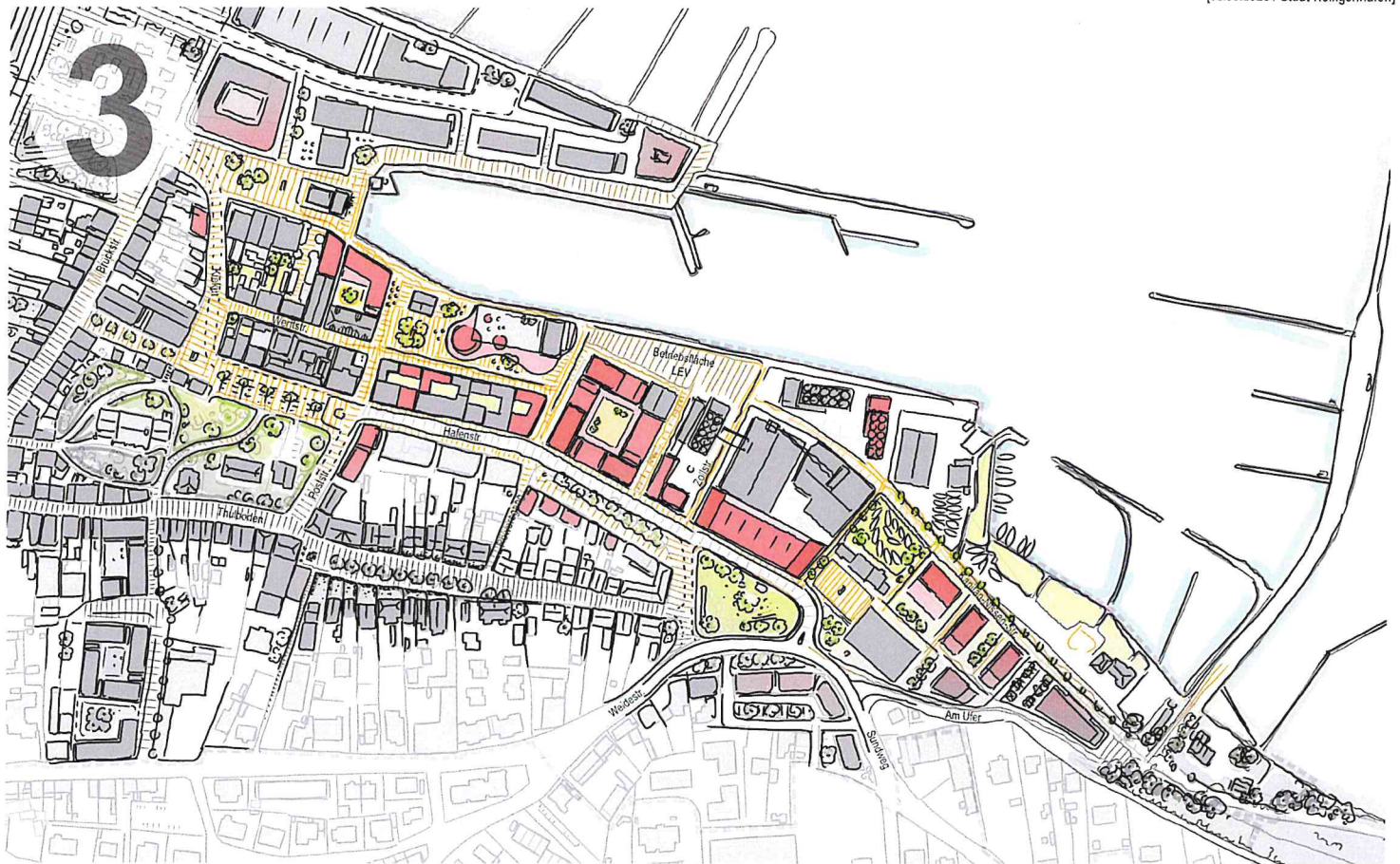
Lageplanskizze o.M.
