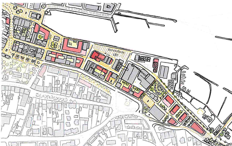
Lageplanskizze Variante
